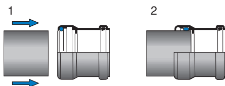
Övergångsmuff MA.
