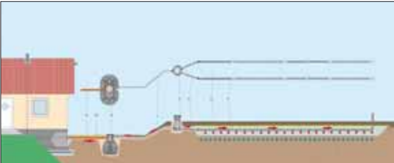
Infiltration med pumpsystem.
