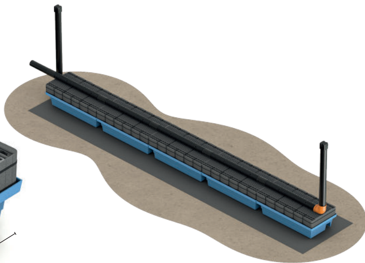
Exempel på infiltration med INDRÄN Plus
