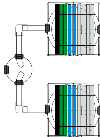
Parallellkopplad BioBox M Sedd ovanifrån med en fördelningsbrunn
