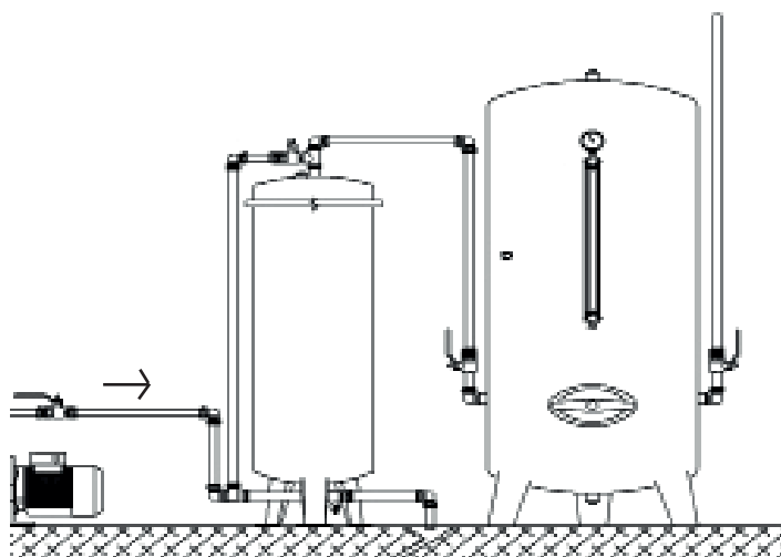
Installationsskiss
