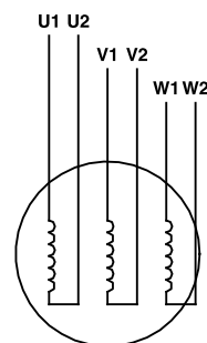
Fig. 17 Oidentifierad kabelmärkning/anslutning – motorer lindade för Y/D-start
