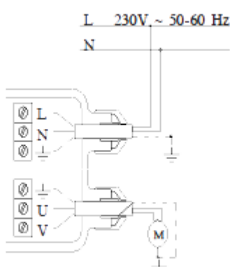
Enfas motorer <1,15kW kopplas enligt ovan.
